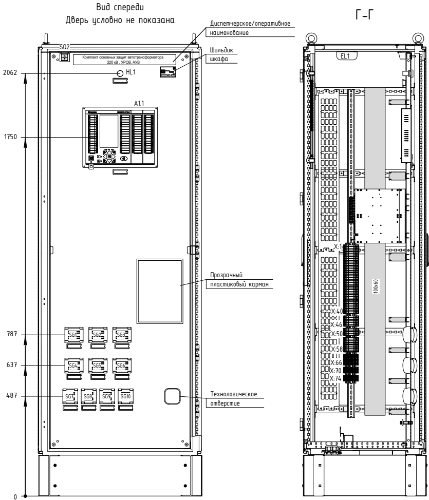
Рисунок В.2 – Чертеж общего вида (часть 2)
